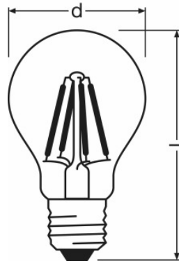
PARATHOM Retrofit CLASSIC A 40 4 W/827 E27 FIL
